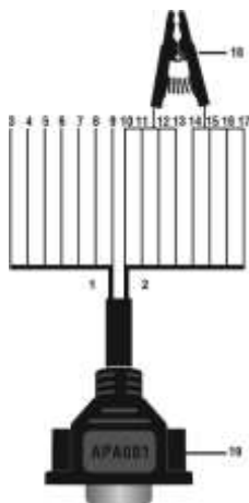
Рисунок 2-4. Кабель MC9S12 с зажимом для микросхем EEPROM
